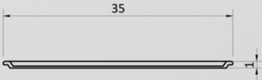
VISTA LATERAL
