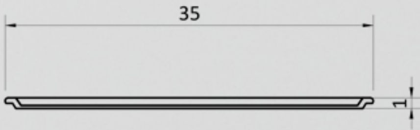
VISTA LATERAL
