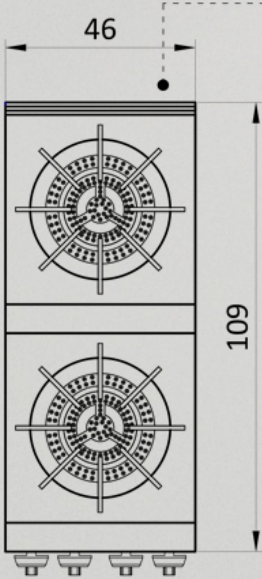
PLANTA
