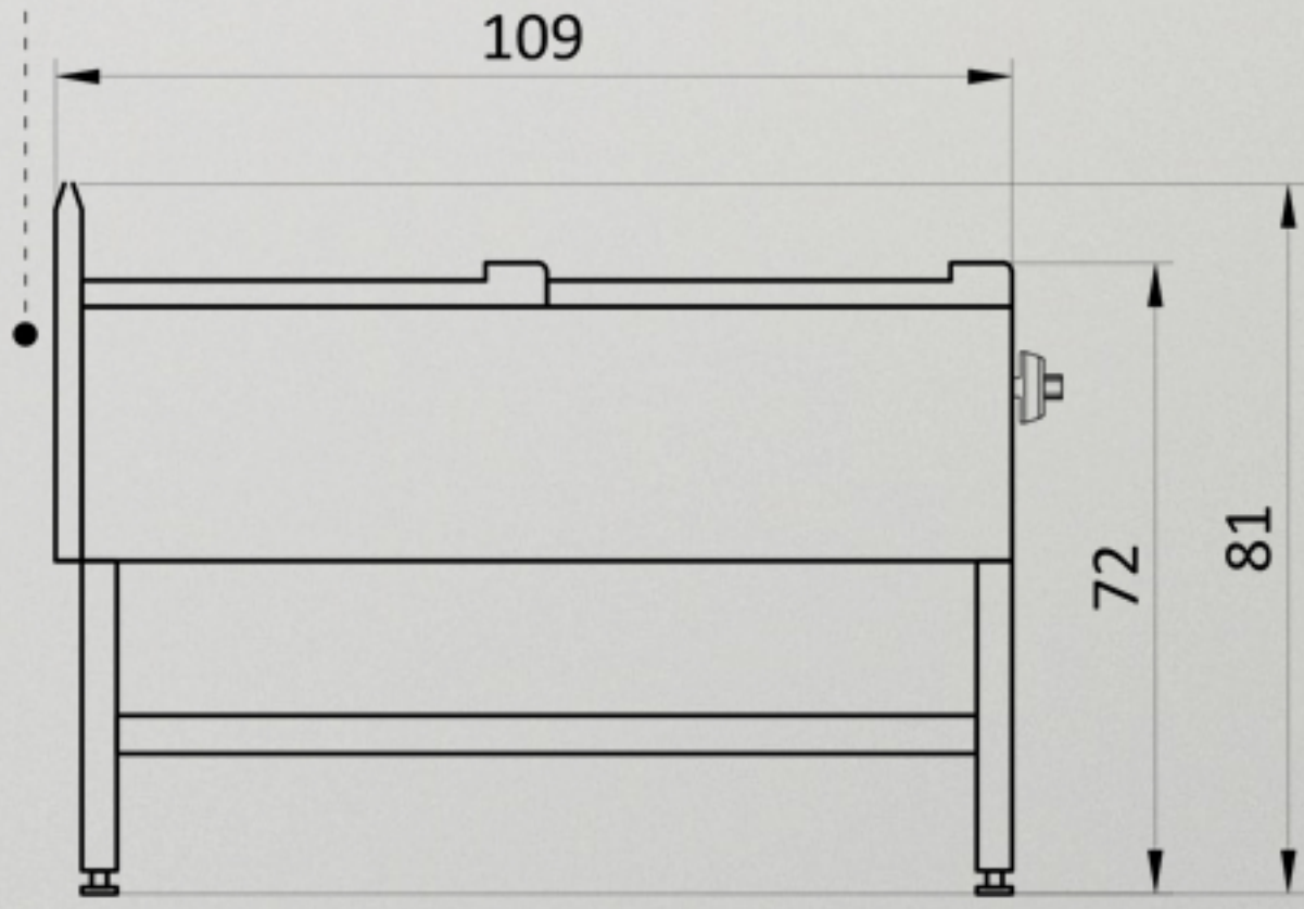
VISTA LATERAL
