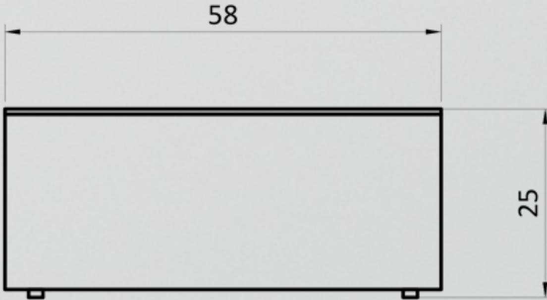
VISTA LATERAL
