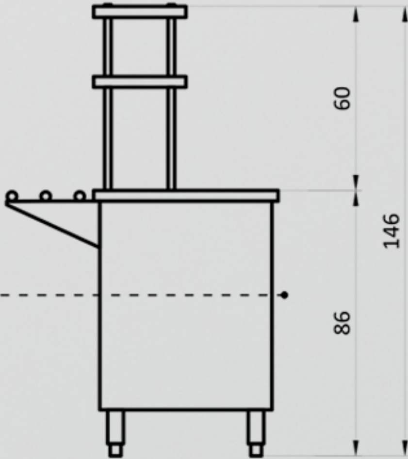
VISTA LATERAL
