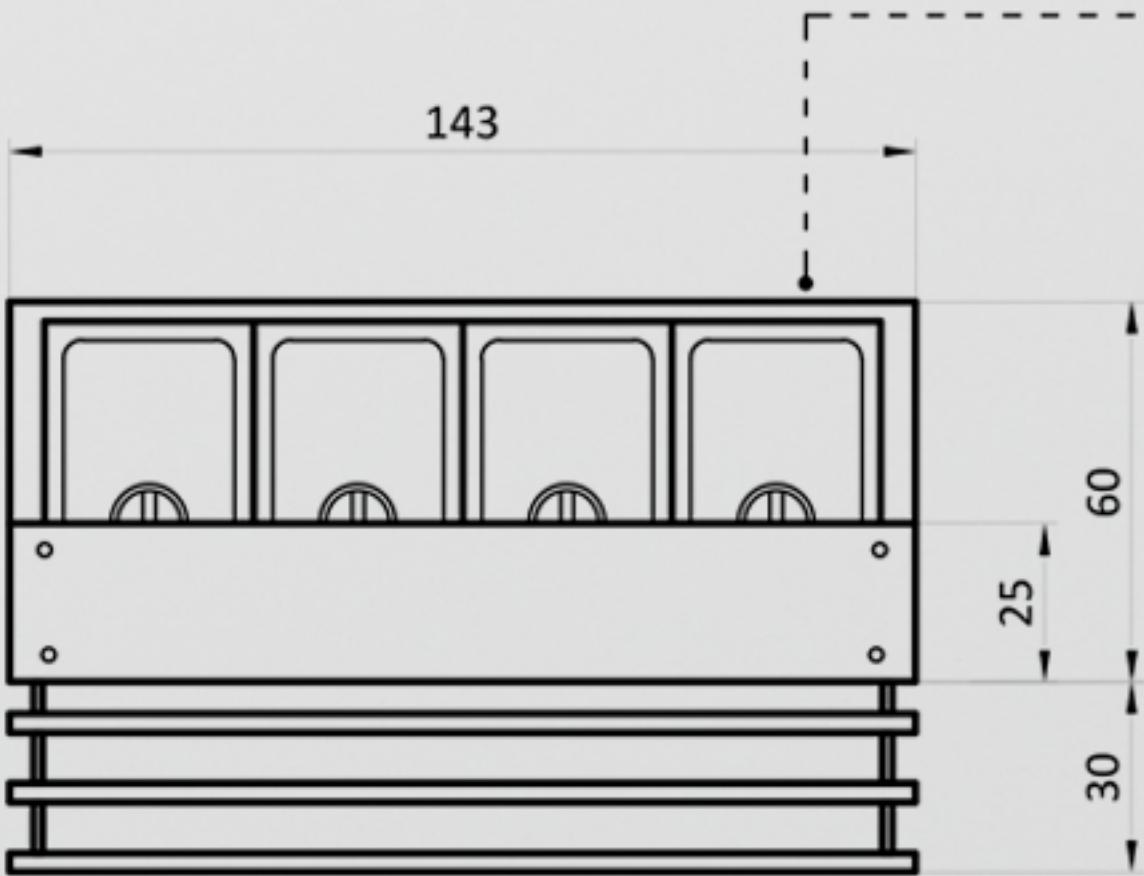
PLANTA
