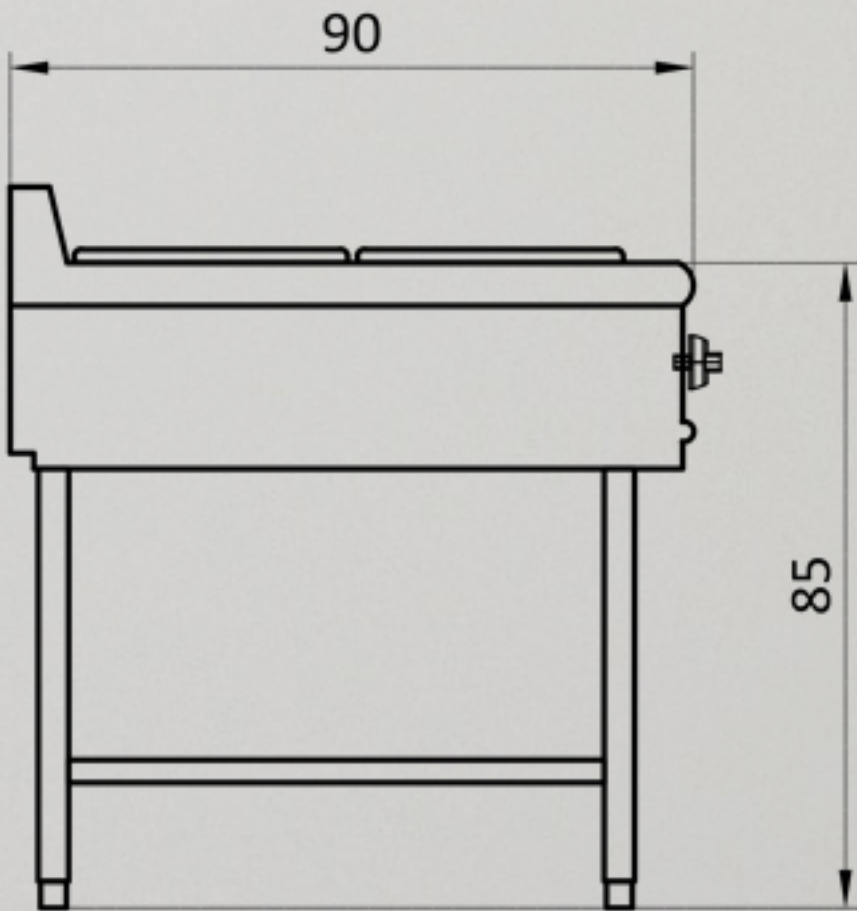
VISTA LATERAL
