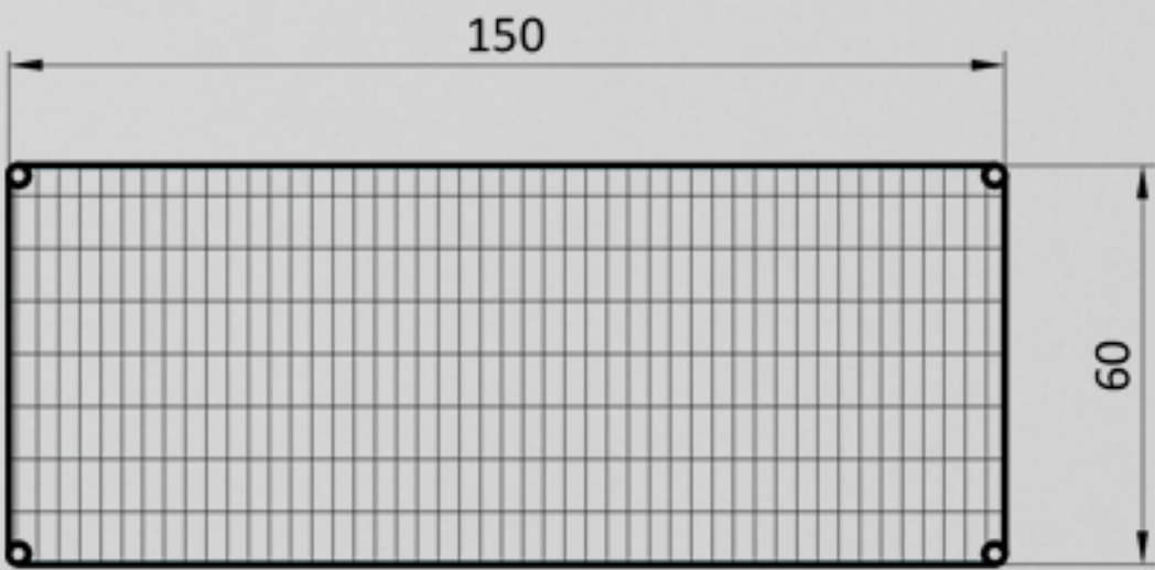
PLANTA
