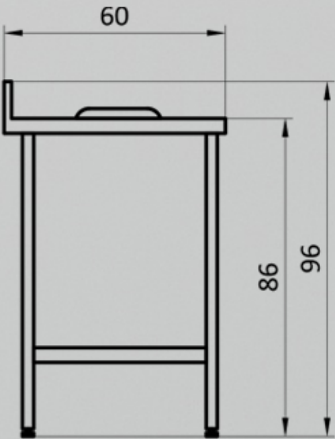
VISTA LATERAL
